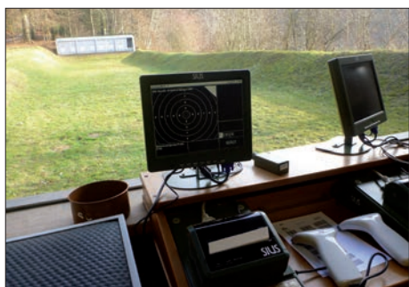
Sicht auf Bedieneinheit der elektronischen Trefferanzeige
